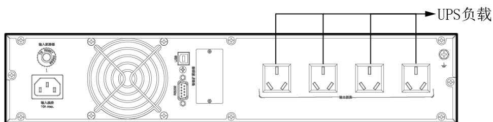
图 4-7 UPS2000-G-2KRTS 输出接线示意图
