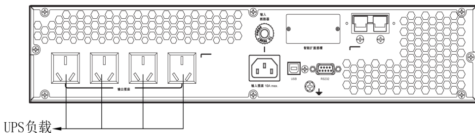
图 4-8 UPS2000-G-2KRTL 输出接线示意图
