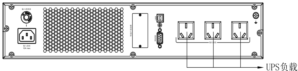
图 4-5 UPS2000-G-1KRTS 输出接线示意图
