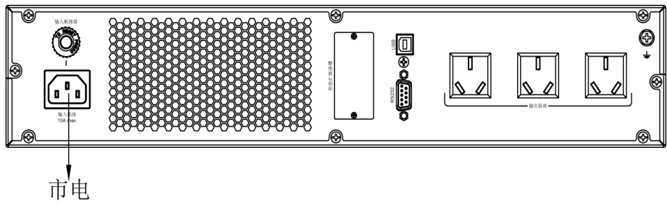
图 4-16 UPS2000-G-1KRTS 输入接线示意图
