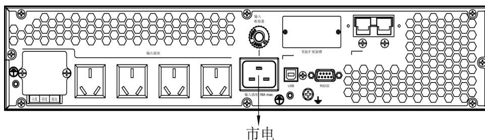
图 4-21 UPS2000-G-3KRTL 输入接线示意图
