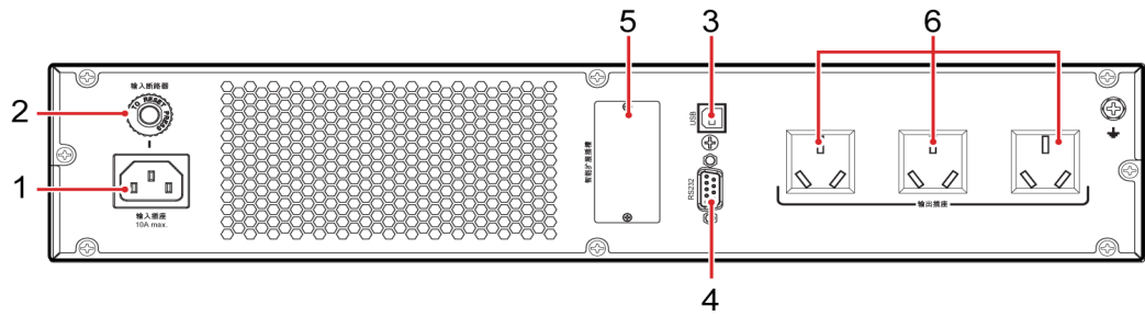
图 2-3 1kVA UPS 标机后视图
