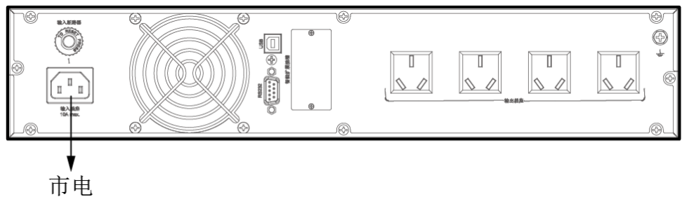
图 4-18 UPS2000-G-2KRTS 输入接线示意图
