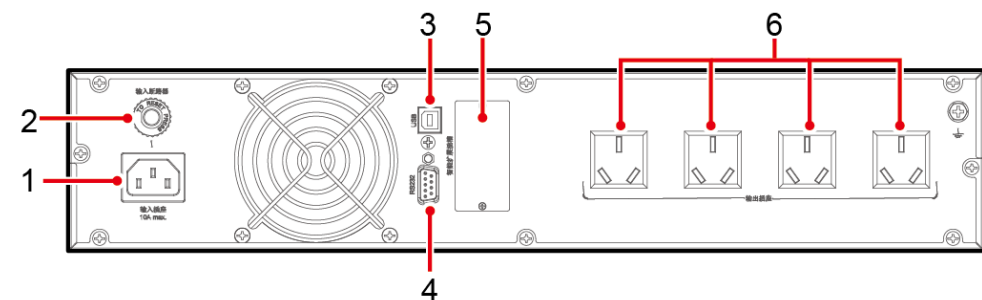
图 2-5 2kVA UPS 标机后视图
