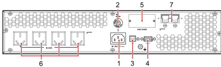
图 2-6 2kVA UPS 长机后视图
