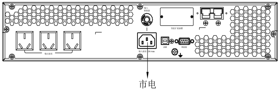
图 4-17 UPS2000-G-1KRTL 输入接线示意图
