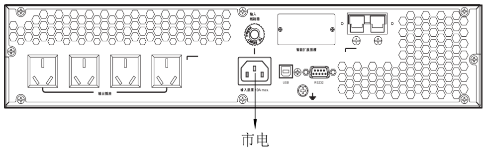
图 4-19 UPS2000-G-2KRTL 输入接线示意图
