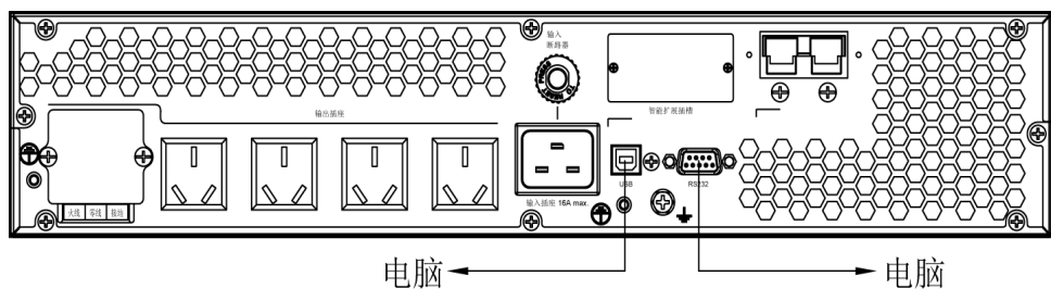
图 4-15 UPS2000-G-3KRTL 通讯线连接示意图
