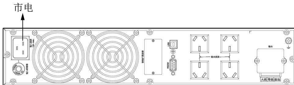
图 4-20 UPS2000-G-3KRTS 输入接线示意图
