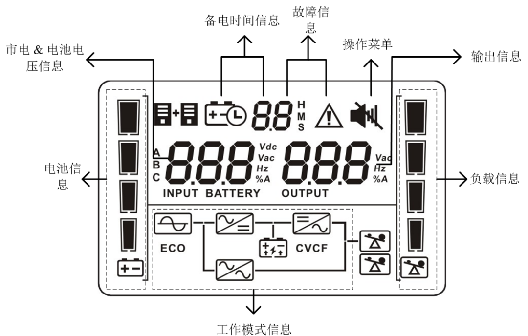
图 5-1 LCD 控制面板
