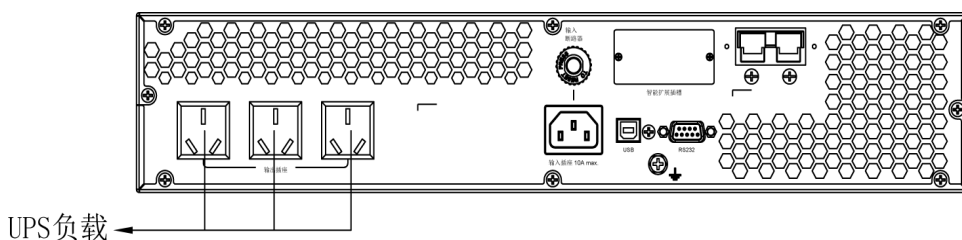
图 4-6 UPS2000-G-1KRTL 输出接线示意图
