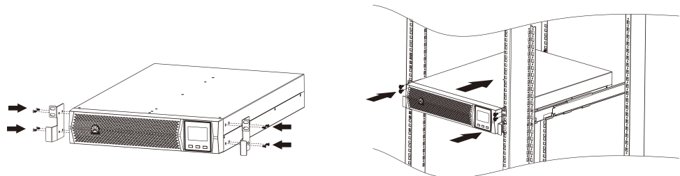
图 4-2 UPS 机架式安装示意图
