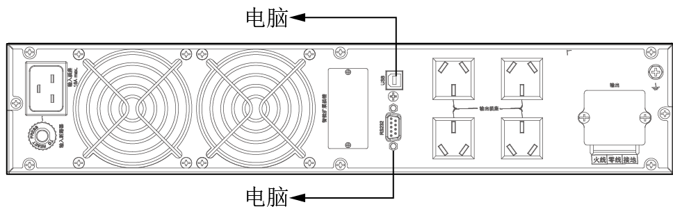
图 4-14 UPS2000-G-3KRTS 通讯线连接示意图
