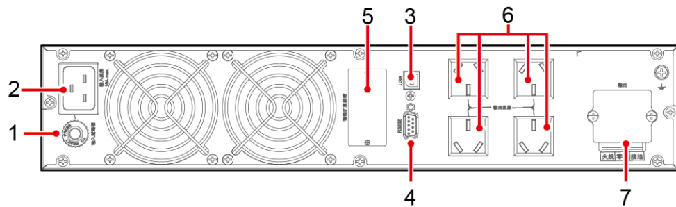
图 2-7 3kVA UPS 标机后视图
