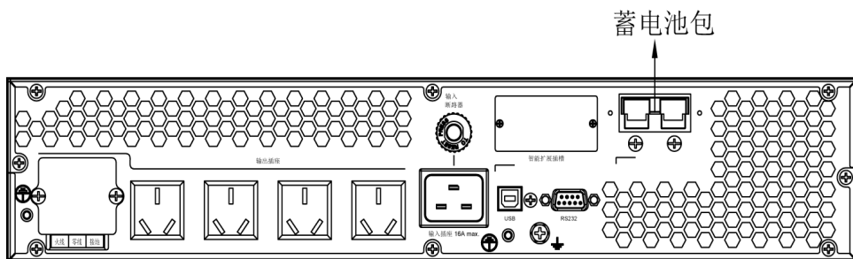
图 4-11 UPS2000-G-3KRTL 电池包接线示意图
