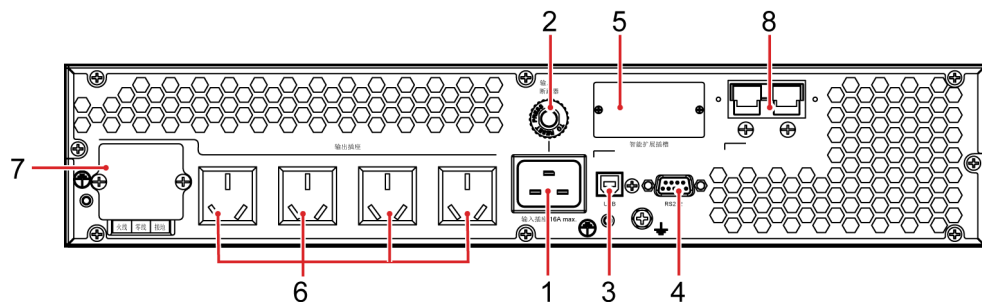
图 2-8 3kVA UPS 长机后视图
