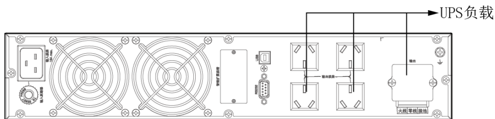
图 4-9 UPS2000-G-3KRTS 输出接线示意图
