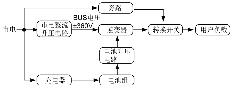
图 2-2 原理框图
