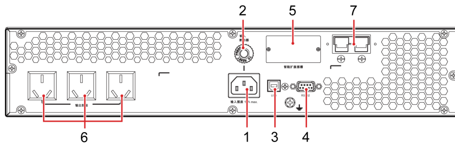
图 2-4 1kVA UPS 长机后视图
