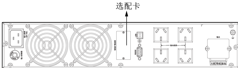
图 4-12 UPS2000-G-3KRTS 选配卡安装位置示意图
