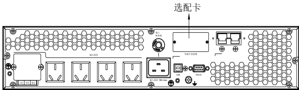
图 4-13 UPS2000-G-3KRTL 选配卡安装位置示意图
