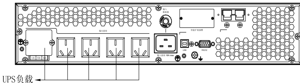
图 4-10 UPS2000-G-3KRTL 输出接线示意图
