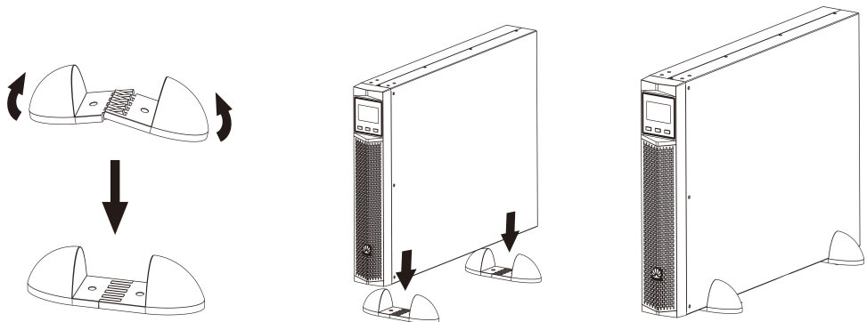
图 4-4 UPS 塔式安装示意图
